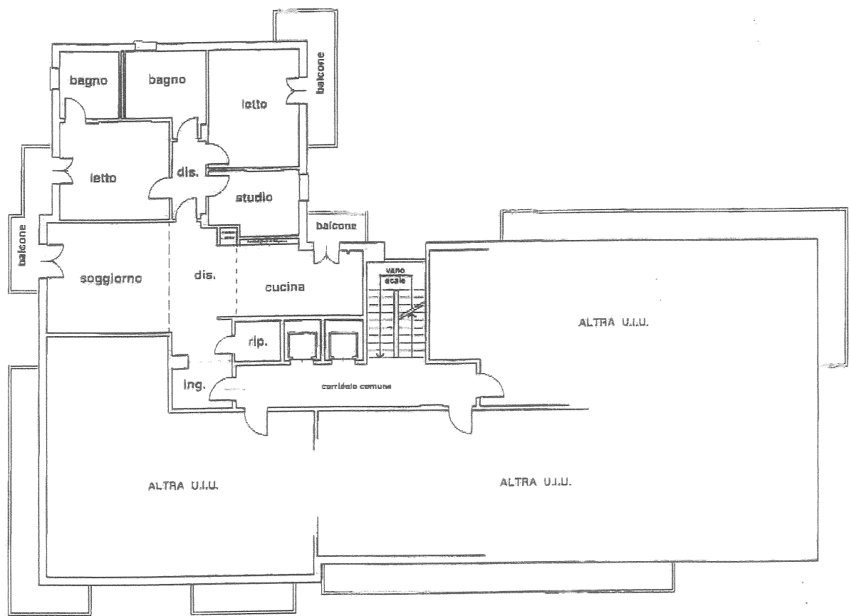
PIANTA PIANO TERZO h = 2,85 ml
